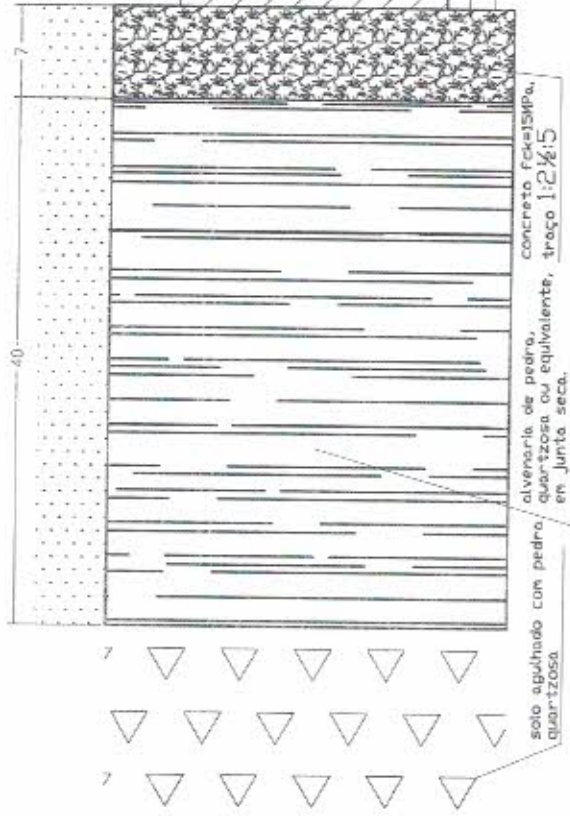
DETALHE DE ALICERCE e CALÇADA
