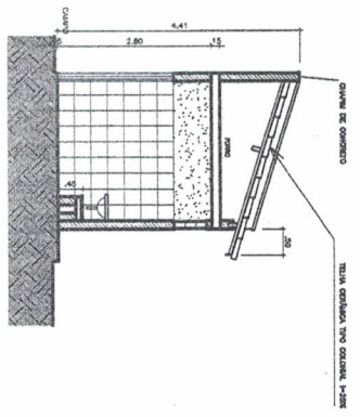
02 CORTE BB ESCALA 1:50
