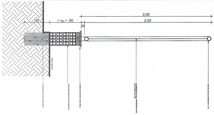
05 CORTE DETALHE MURETA ESCALA 1:10
