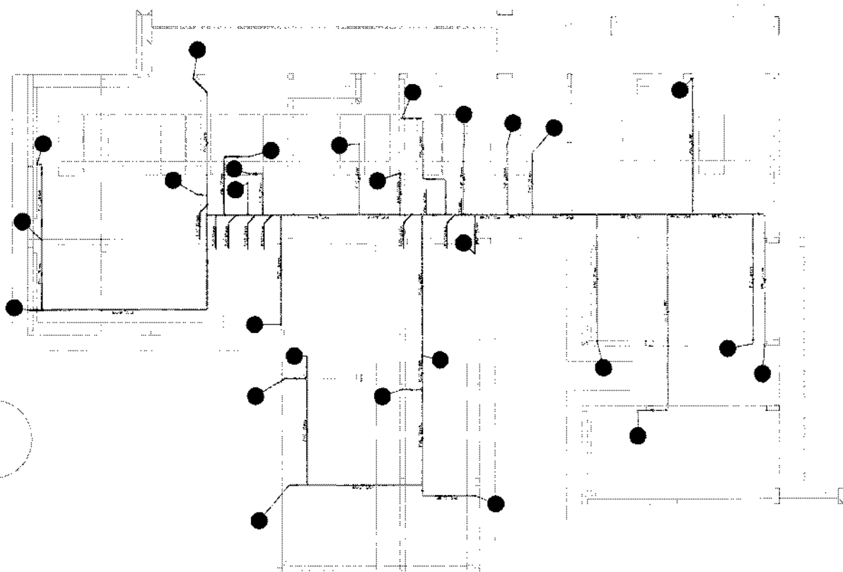
PLANTA - HIDRÁULICO - COBERTURA ESC. 1/50
